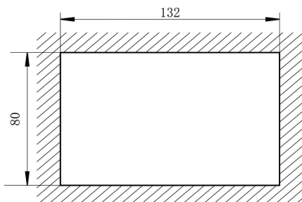
开孔尺寸图
