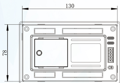
正视图
